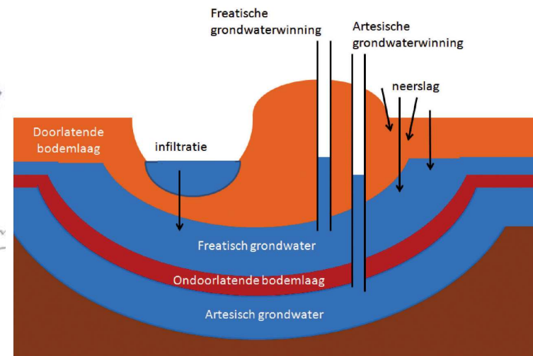
Figuur 3.3 - Grondwaterwinning voor de drinkwatervoorziening
